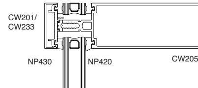
① HEADER
