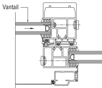
Accrochage réciproque
