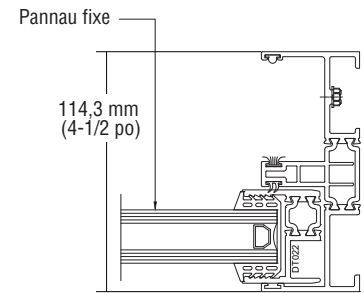
Montant fixe
